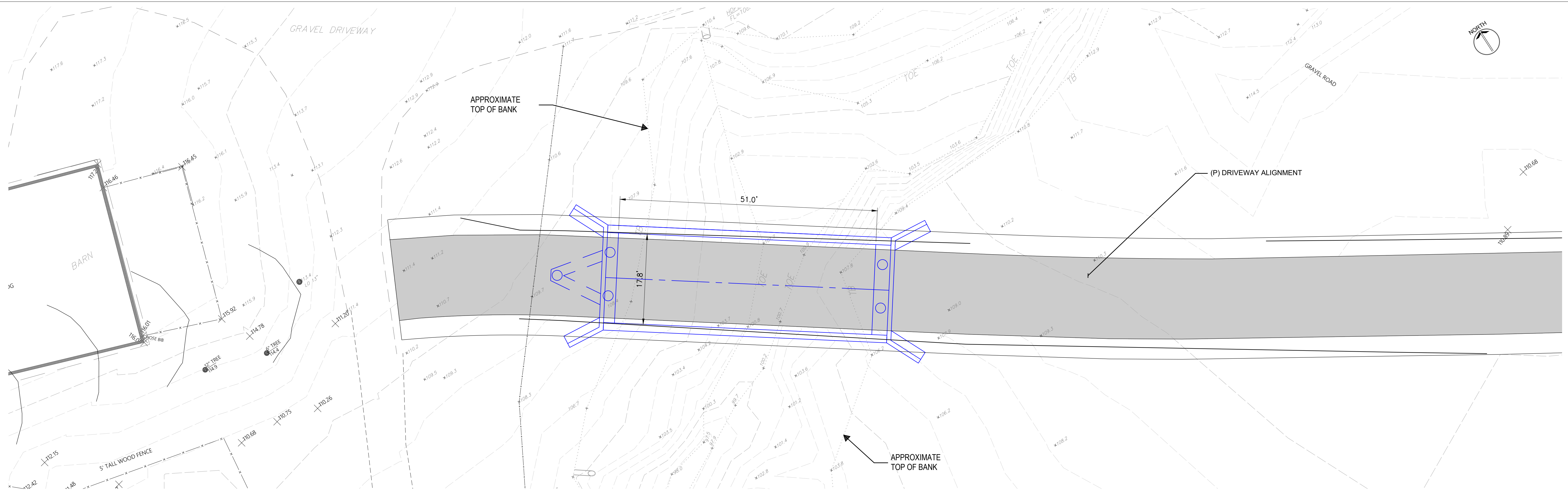
PLAN SCALE: 1"=10'
